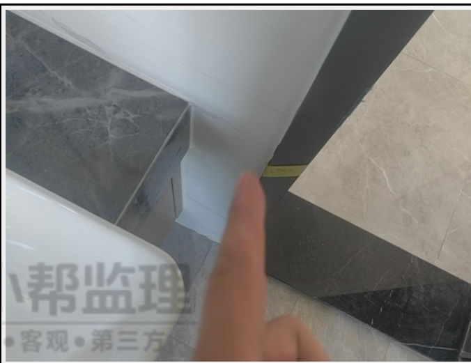
2、合金门内测打胶不均
